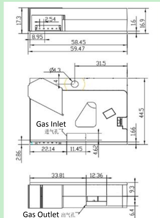
Fig1.Structure
